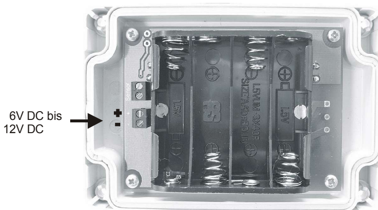
Abbildung 4: Anschluss des Netzteil
