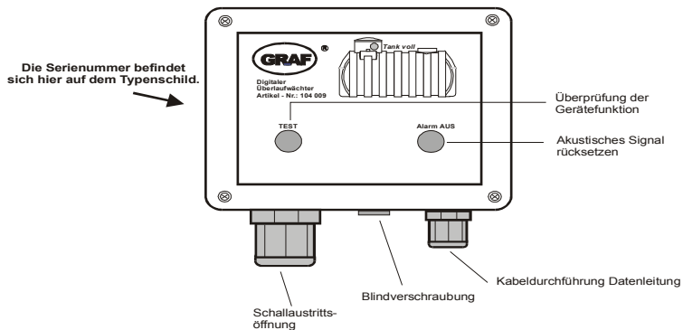
Abbildung 1: Geräteübersicht
