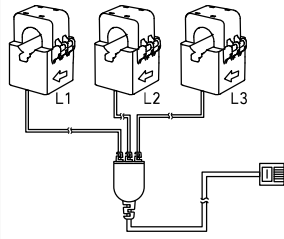
Stromwandler
