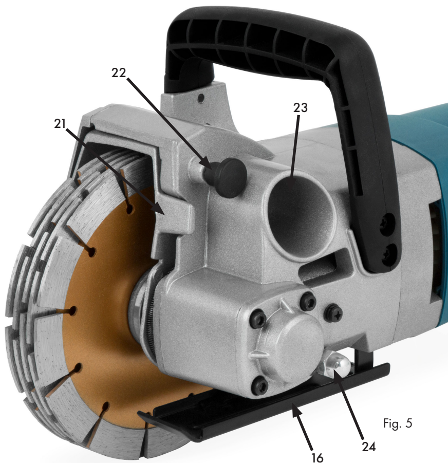
La Figura 5 mostra la testa di taglio con il cofano di protezione represso.
