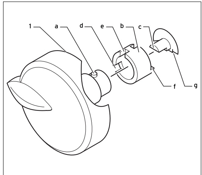
Afb. 5.3 Temperatuurkeuzeknop
