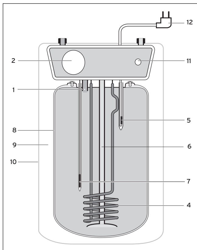
Fig. 3.1 Schéma de fonctionnement VEN U
