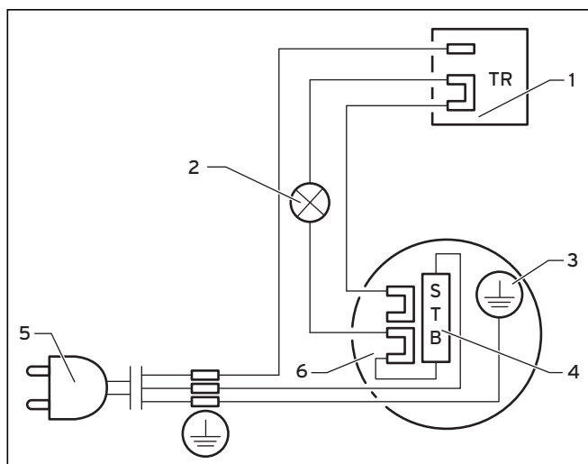
Afb. 4.8 Schakelschema
