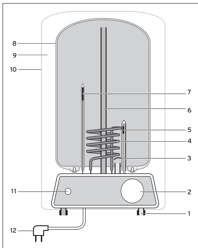
Afb 3.2 Functieschema VEN O
