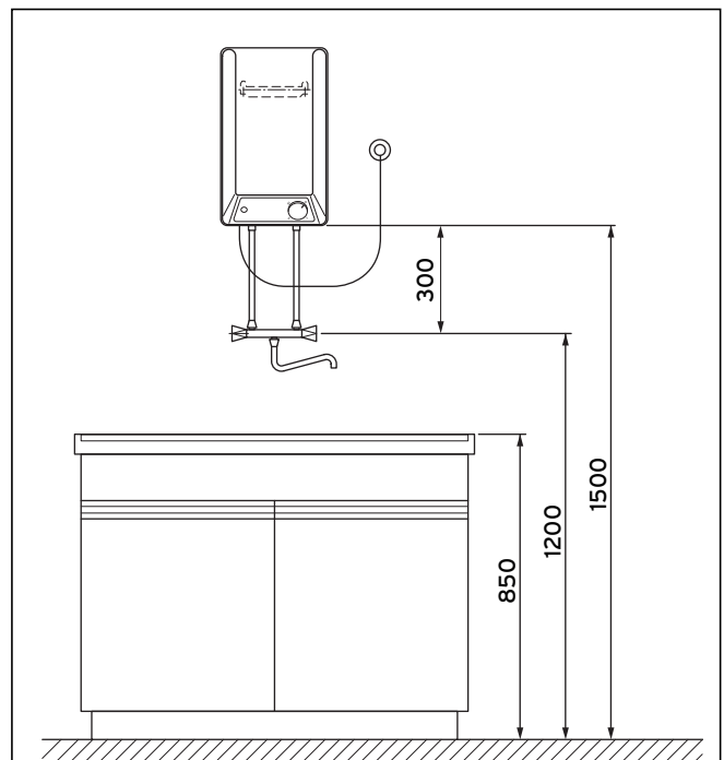
Sl. 4.5 Primjer instalacije VEN 10/5 O
