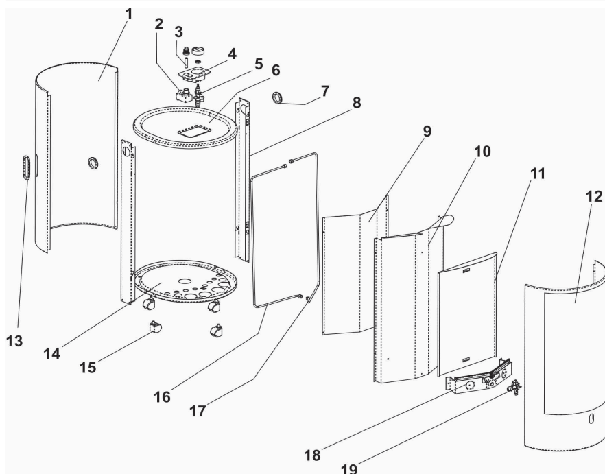
Abb. 6a: Explosionszeichnung
