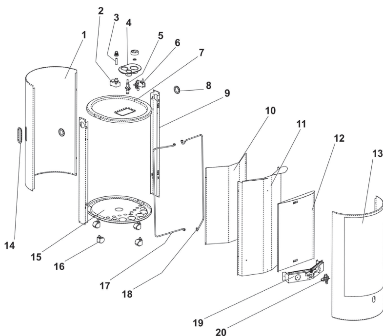
Abb. 6b: Explosionszeichnung
