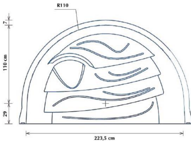
Vorderansicht
