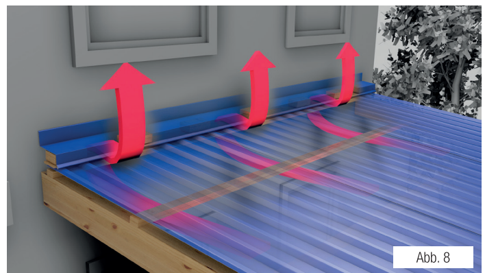
Ein hinterlüfteter Wandanschluss sorgt für den nötigen Luftaustritt, damit sich die Kondensatbildung verringert.
