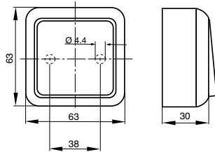
Schalter-/Steckdosenkombination 2)
