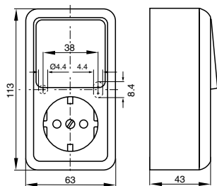
Schalter-/Steckdosenkombination 2)
