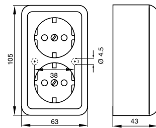
Steckdose 2-fach 2)
