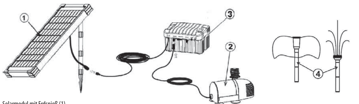
Solarmodul mit Erdspeiß (1) Solarpumpe mit 5 m Anschlussleitung (2) Akku-Batterie mit 5 m Anschlussleitung (3) 4 Steigrohr und 2 Wasserdüsen (4)
