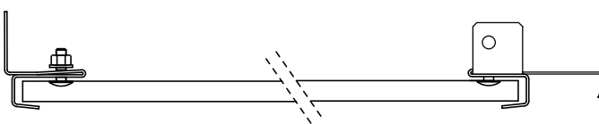
Kopfprofil Rückwand top frame profile back wall profil de tête paroi arrière kopprofiel achterwand
