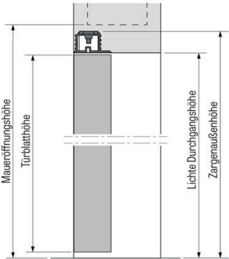
Seitenansicht - Öffnungsrichtung Drücken
