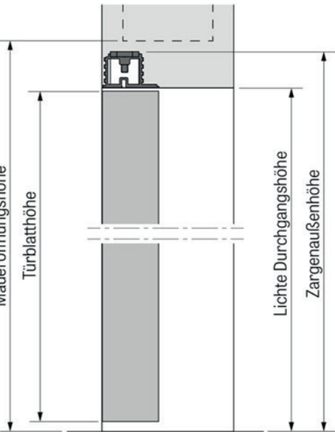
Seitenansicht - Öffnungsrichtung Drücken
