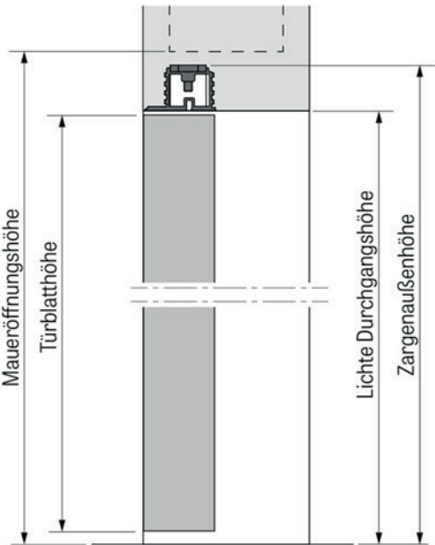
Seitenansicht - Öffnungsrichtung Ziehen
