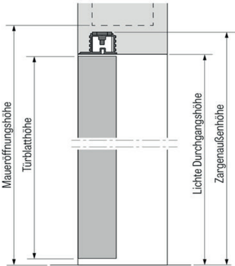
Seitenansicht - Öffnungsrichtung Ziehen
