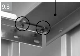
Kopfprofil Vorderwand | top section, front wall profil de tête paroi avant | kopprofiel voorwand
