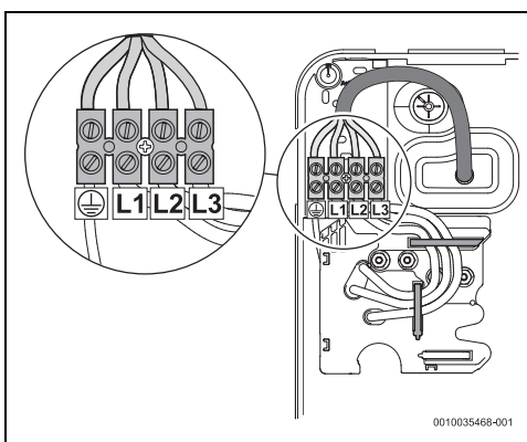
Fig. 42 Raccord supérieur
