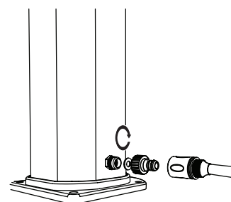
4 Raccorder le tuyau d'eau (eau froide) à l'entrée d'eau de la douche
